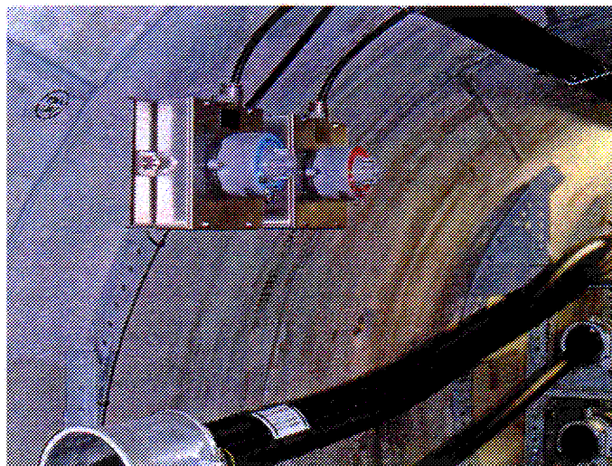
ガスセンサの洞道内設置状況 (酸素センサと可燃性ガスセンサ)
