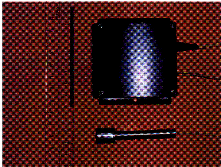
上：電磁石型光センサ外観 下：ファラデー素子型光センサ外観
